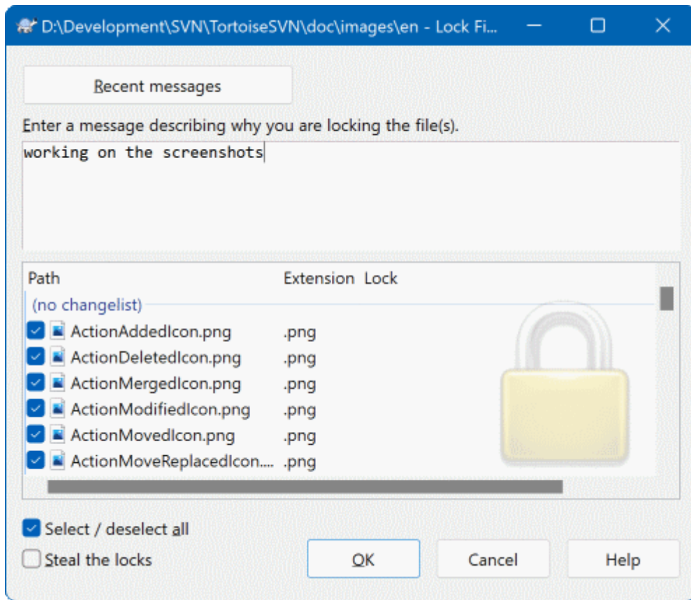
图 4.59. 锁定对话框
