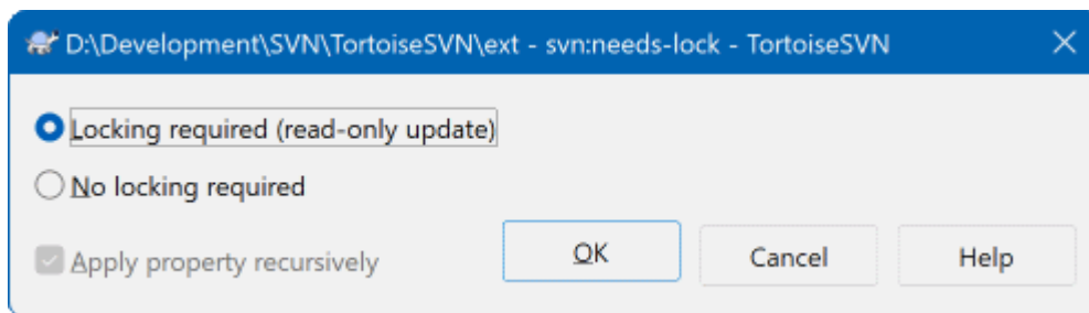
图 4.49. svn:needs-lock 属性页
