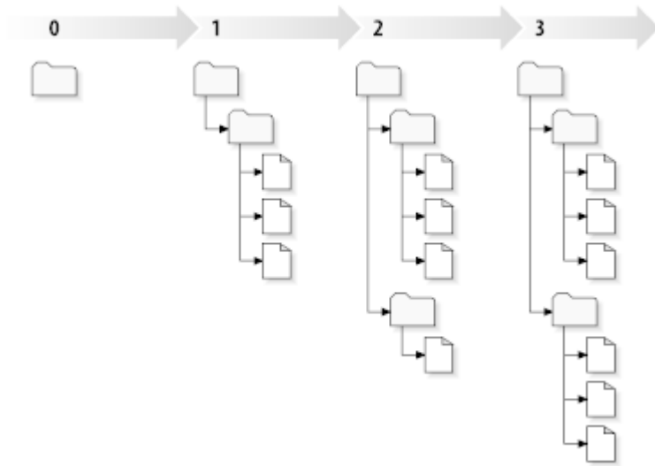
图 2.7. 版本库
