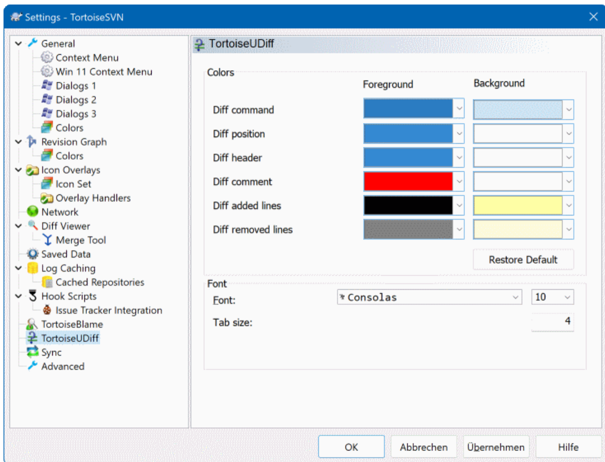
Рисунок 4.92. Диалог Настройки, страница TortoiseUDiff
