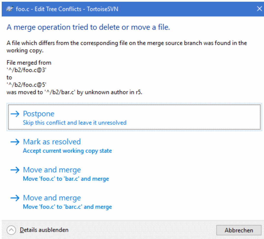
Рисунок 4.58. The Merge Tree Conflict Dialog
