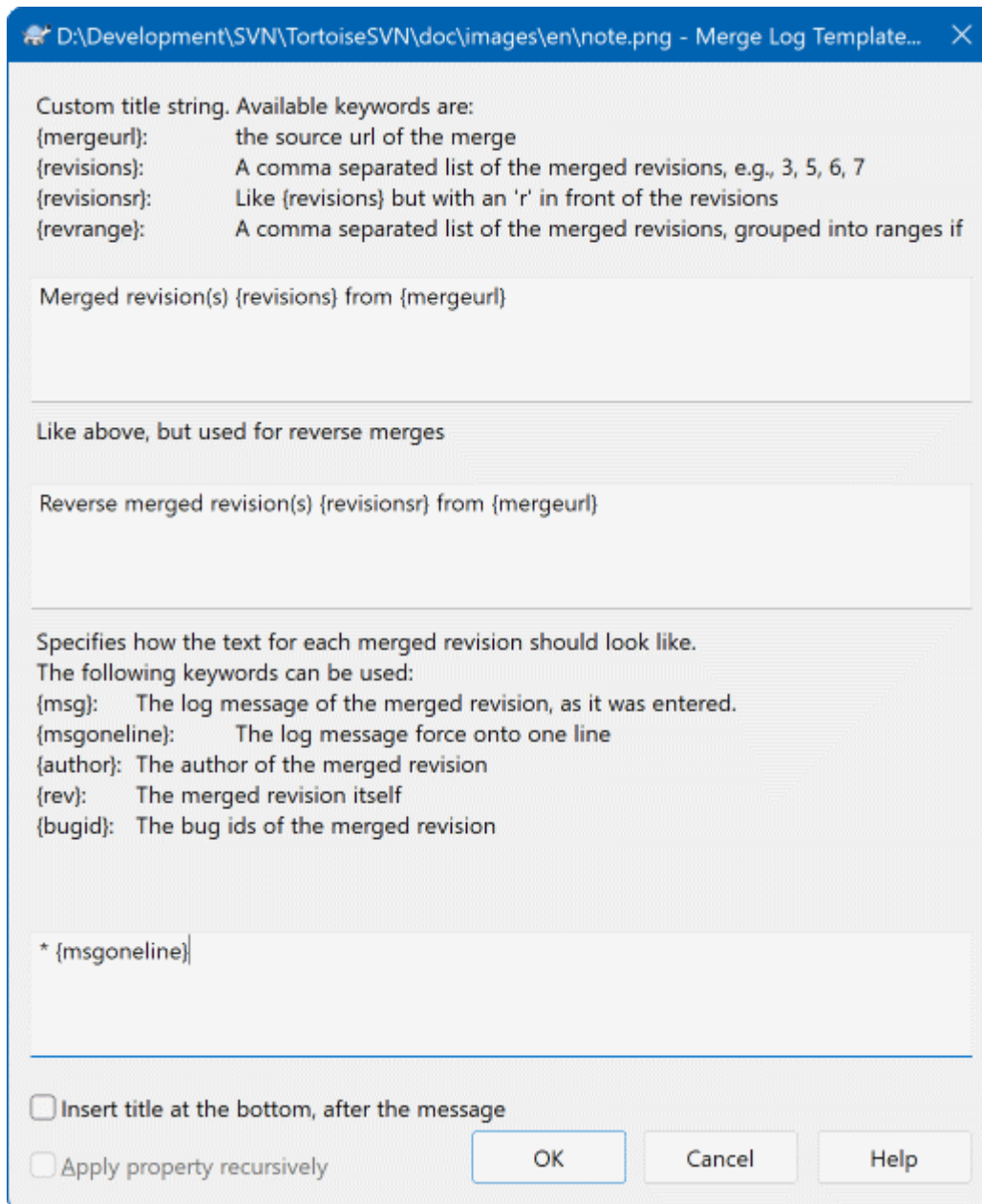
Рисунок 4.52. Диалог свойства шаблонов сообщения журнала для слияния
