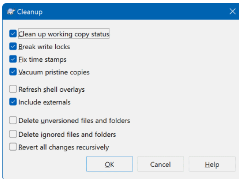
Рисунок 4.36. Диалог Очистки
