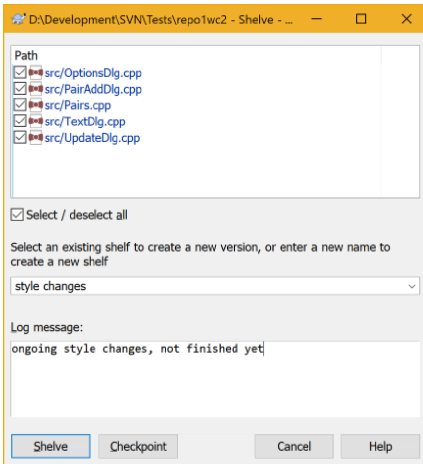
Рисунок 4.16. Shelve dialog
