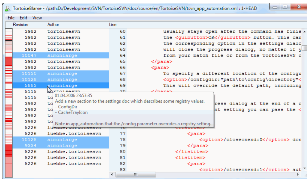
Figura 4.61. TortoiseBlame
