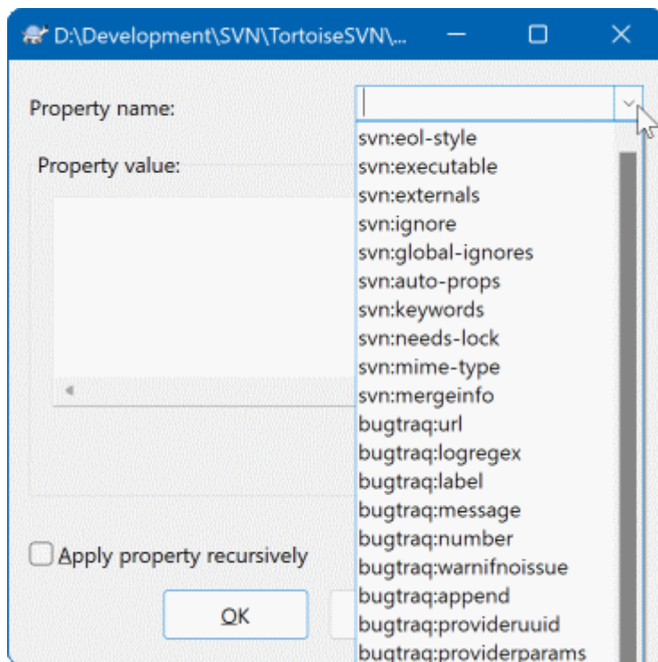
Figura 4.38. Añadiendo propiedades
