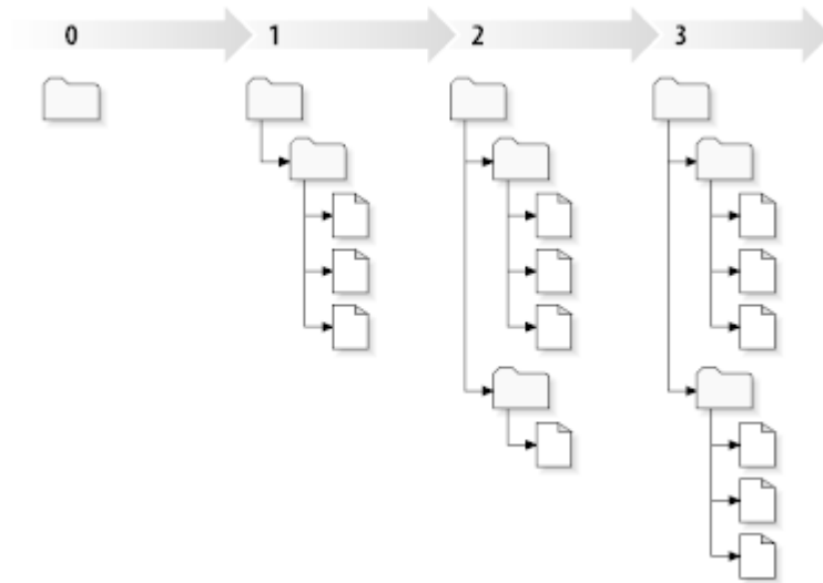
Figura 2.7. El repositorio
