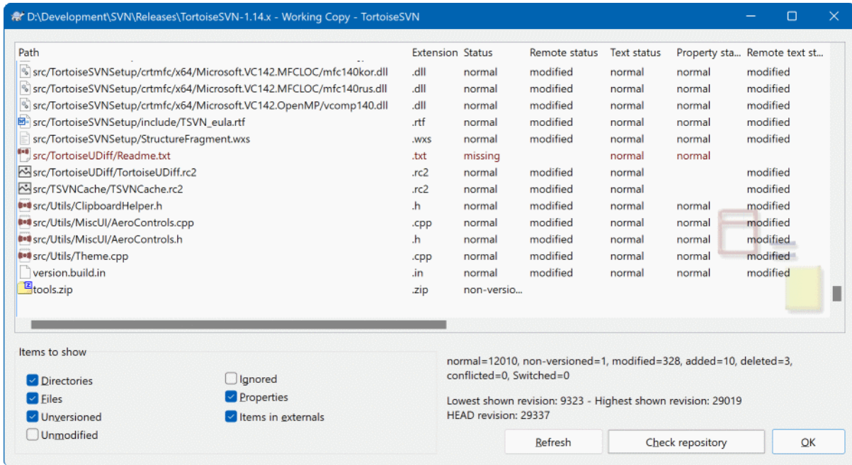
Figura 4.14. Comprobar modificaciones
