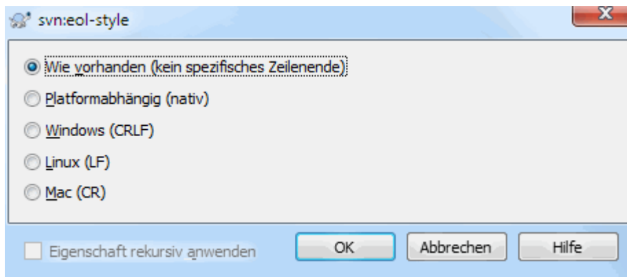
Abbildung 4.43. Eigenschaftsseite svn:eol-style
