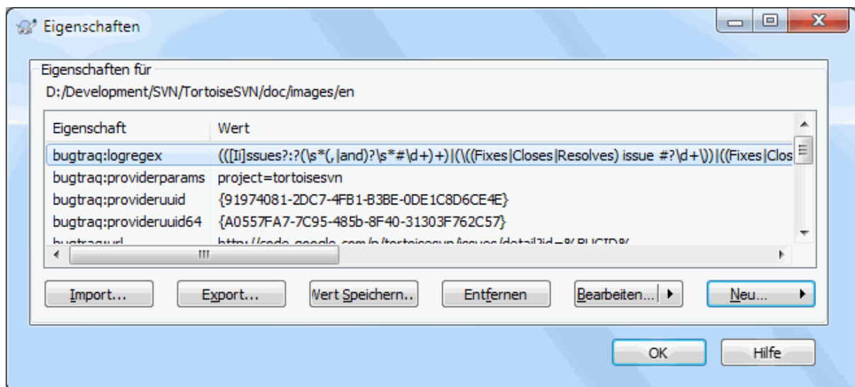
Abbildung 4.37. Subversion-Eigenschaftsseite
