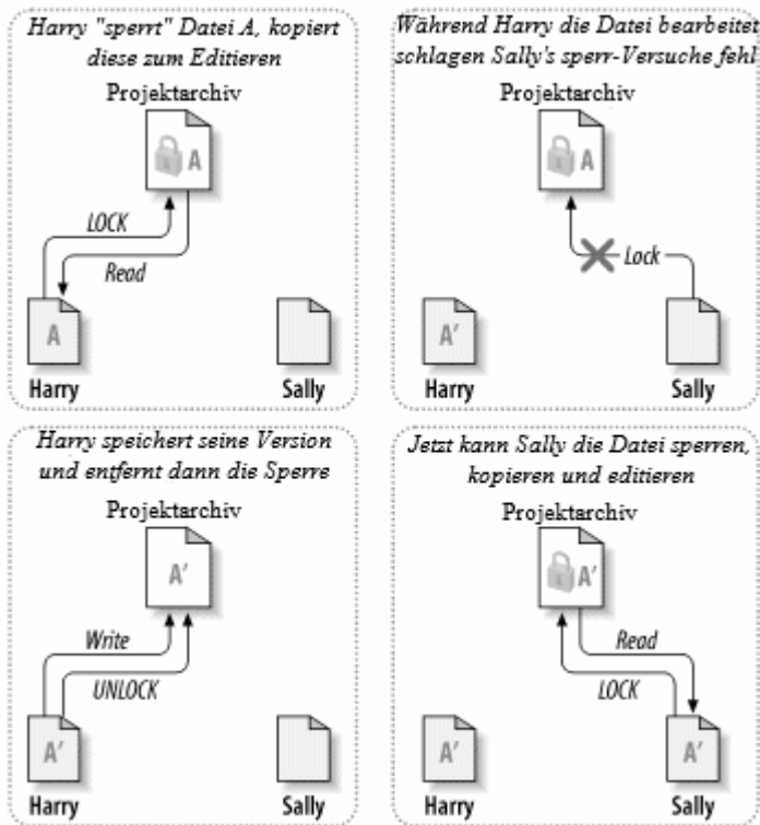
Abbildung 2.3. Die Sperr-Ändern-Freigeben-Lösung
