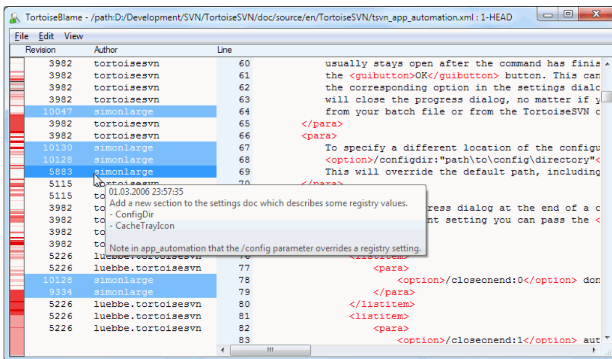
Slika 4.64. TortoiseBlame
