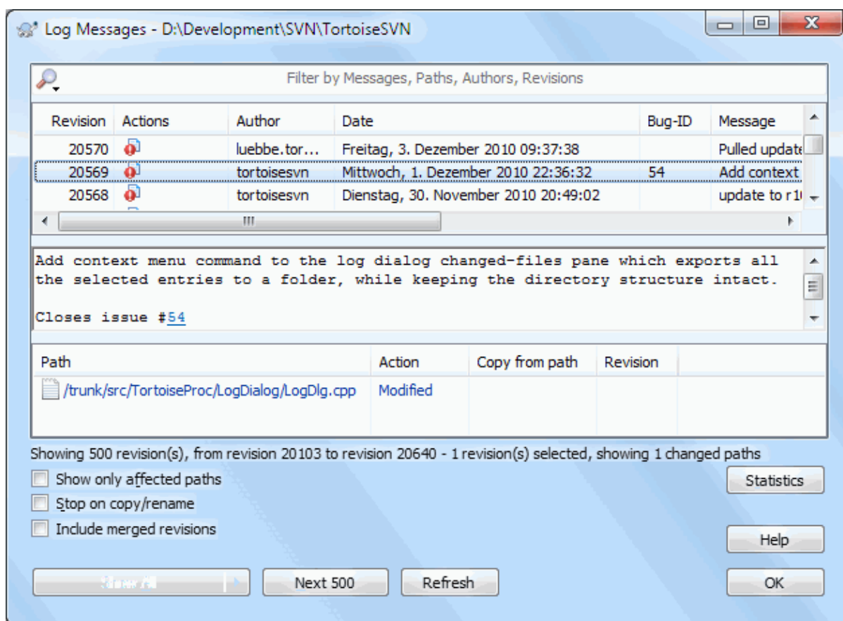
Slika 4.18. Okno dnevnika
