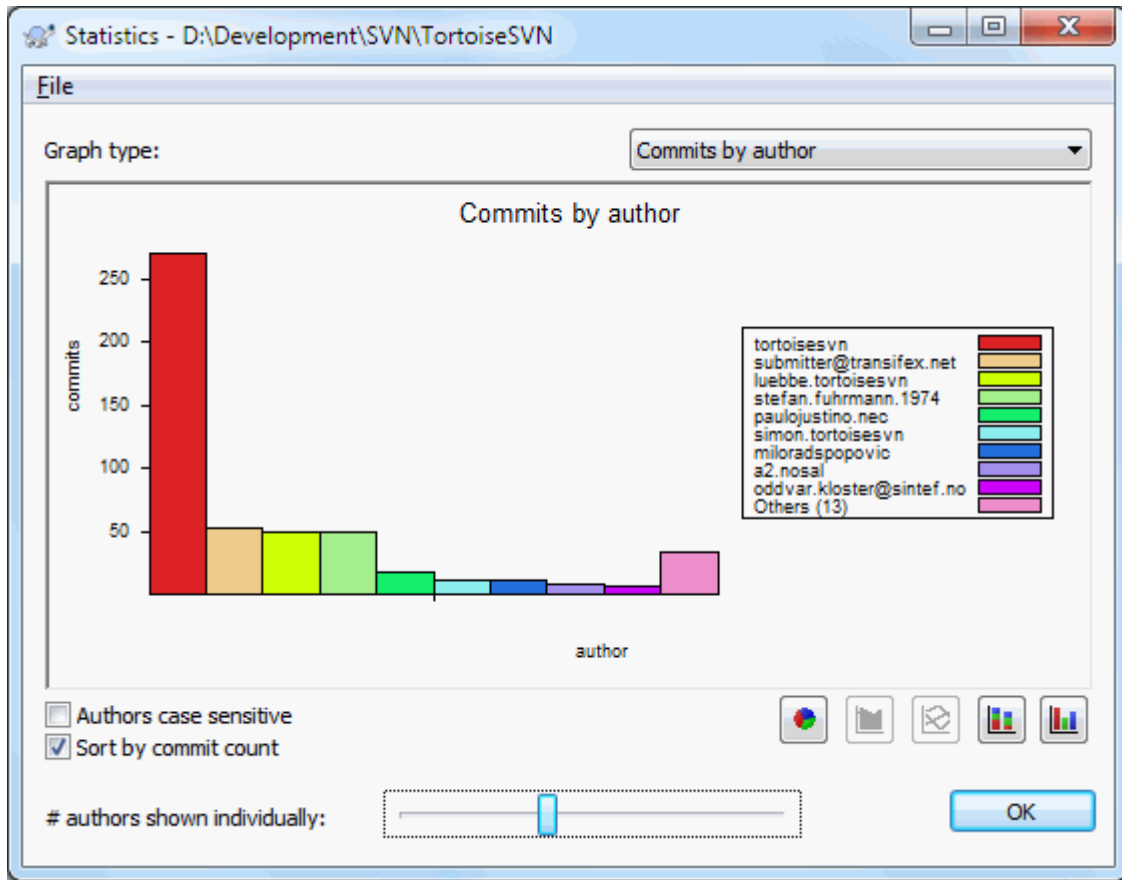
图 4. 25. 作者提交次数统计柱状图
