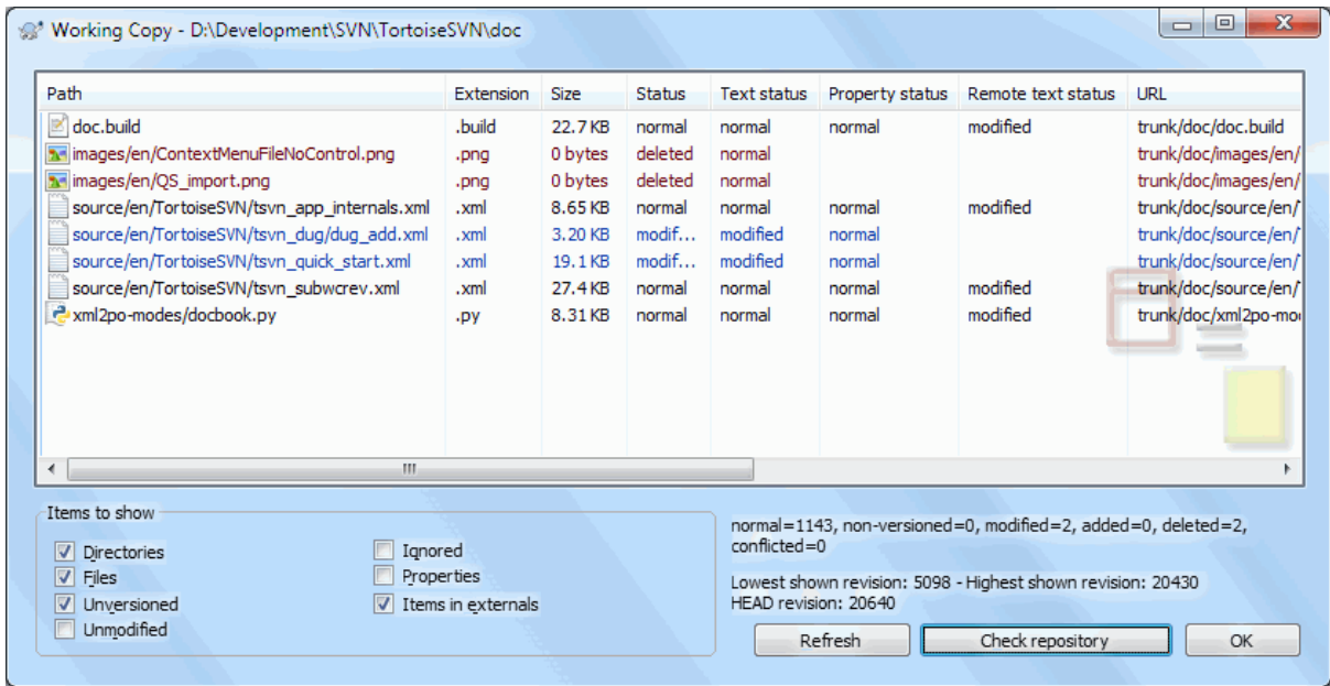
图 4.61. 检查修改对话框
