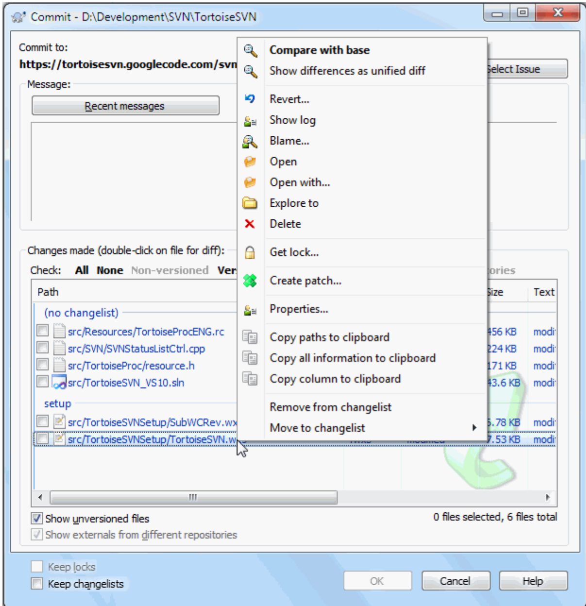
图 4.8. 提交对话框
