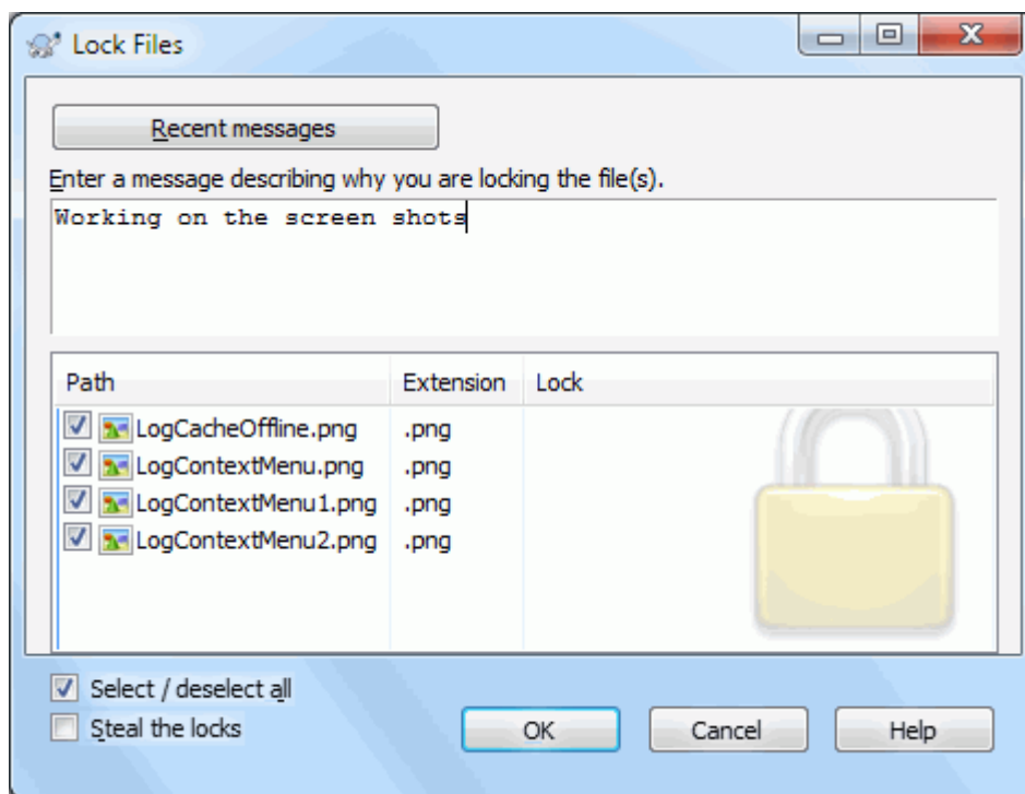
图 4.60. 锁定对话框
