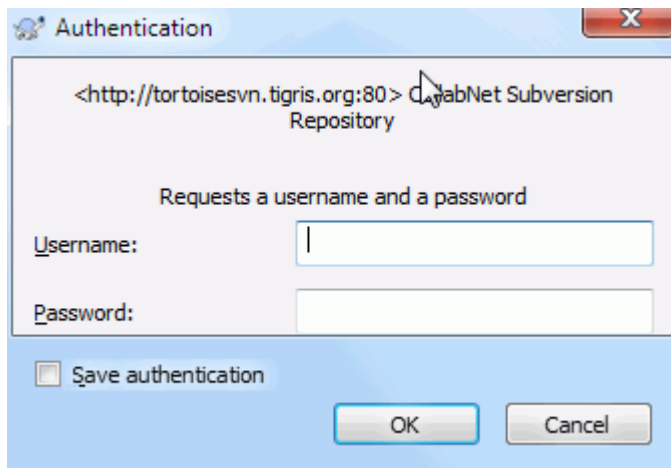
图 4.5. 认证对话框
