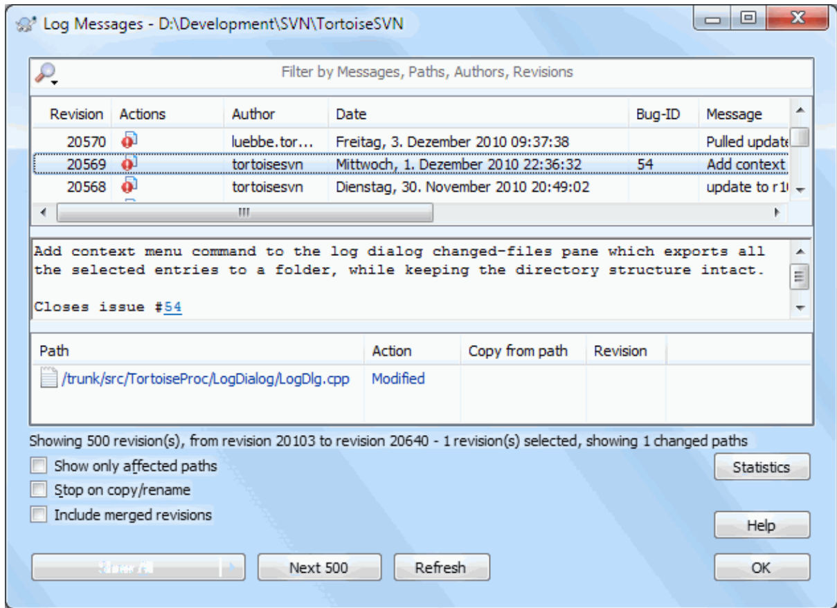
图 1.4. 日志对话框
