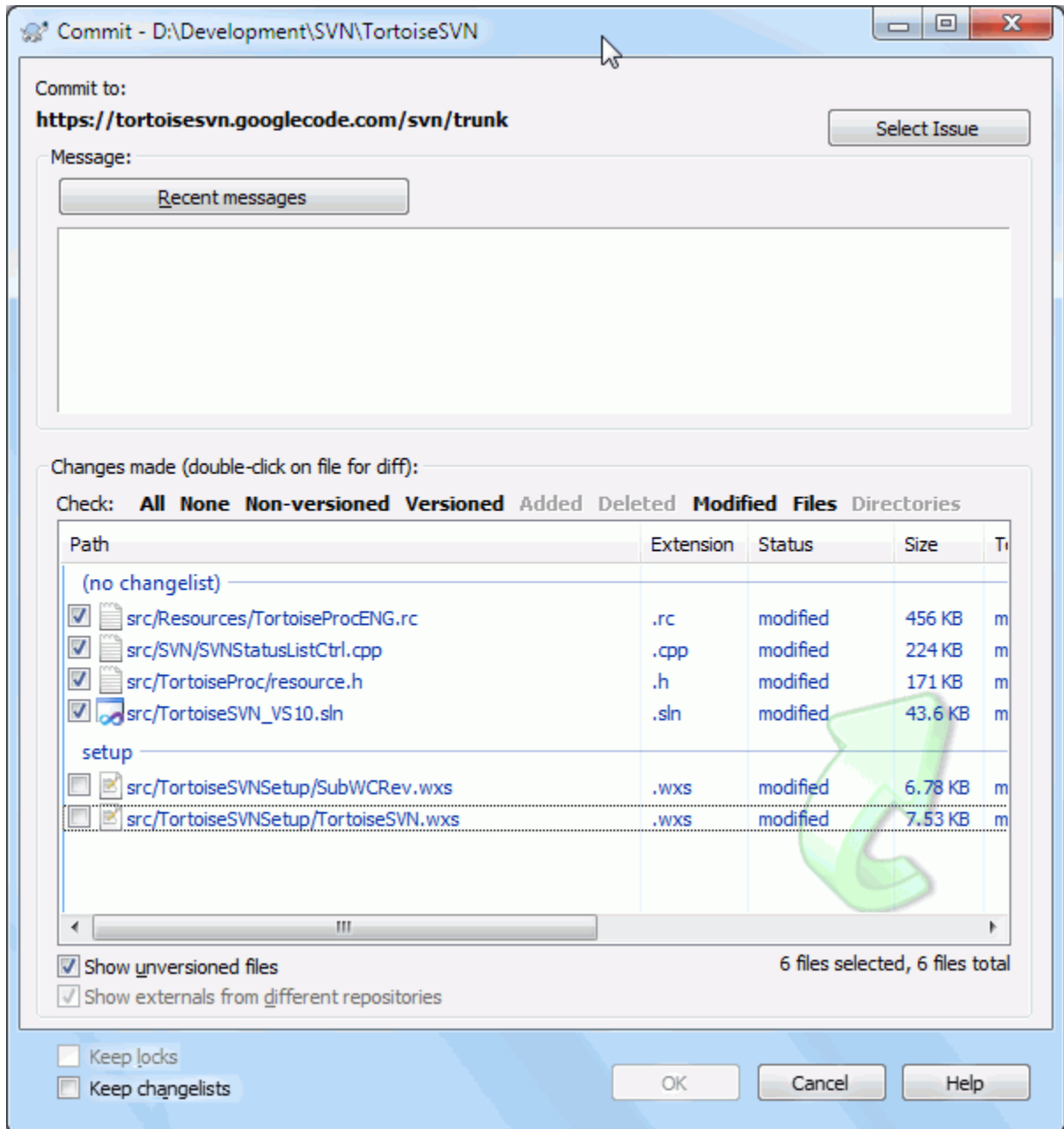
图 4.15. 带有修改列表的提交对话框
