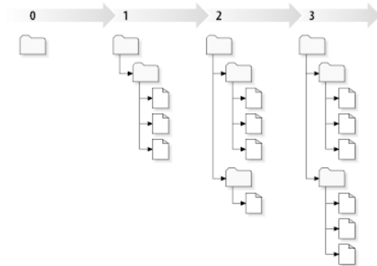
图 2.7. 版本库
