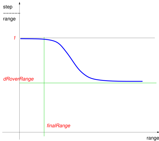
Fig. 8.1: Step limit.
