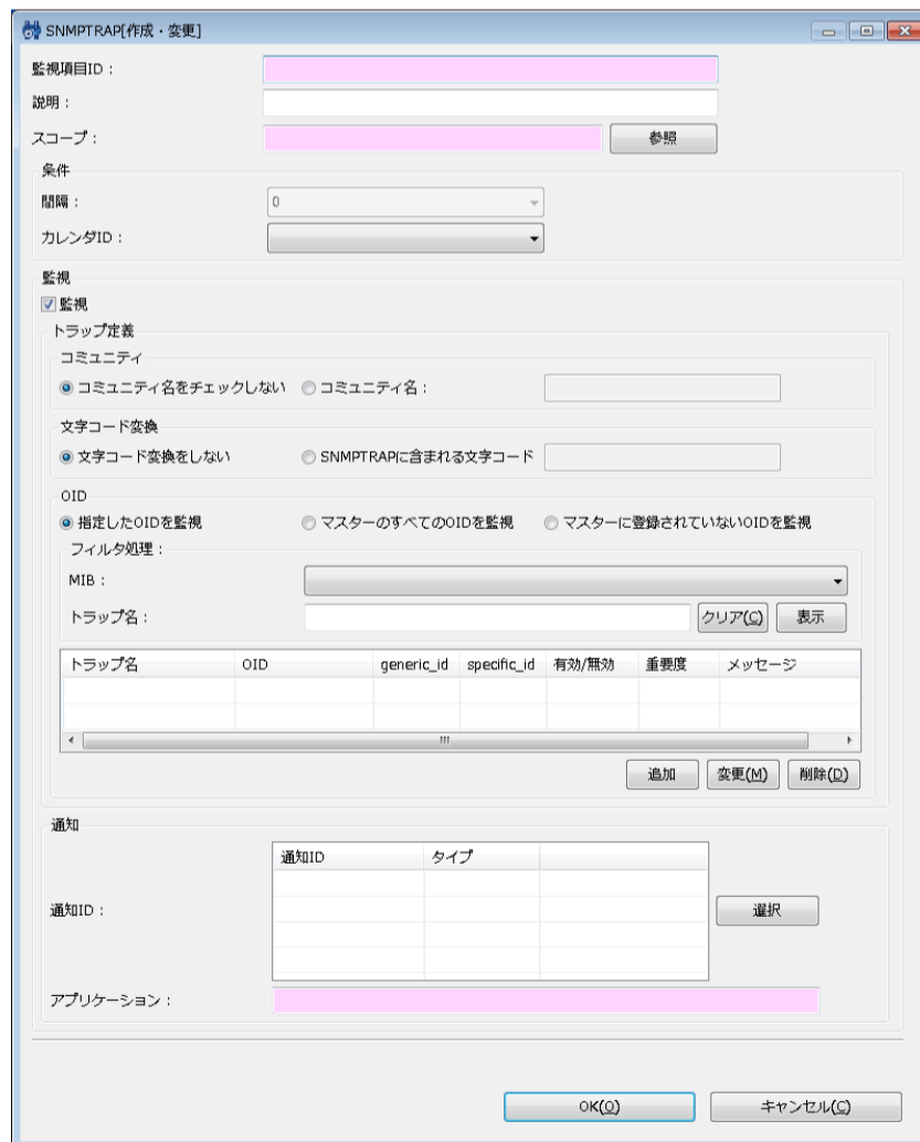
図 7-13 SNMPTRAP[作成・変更]ダイアログ
