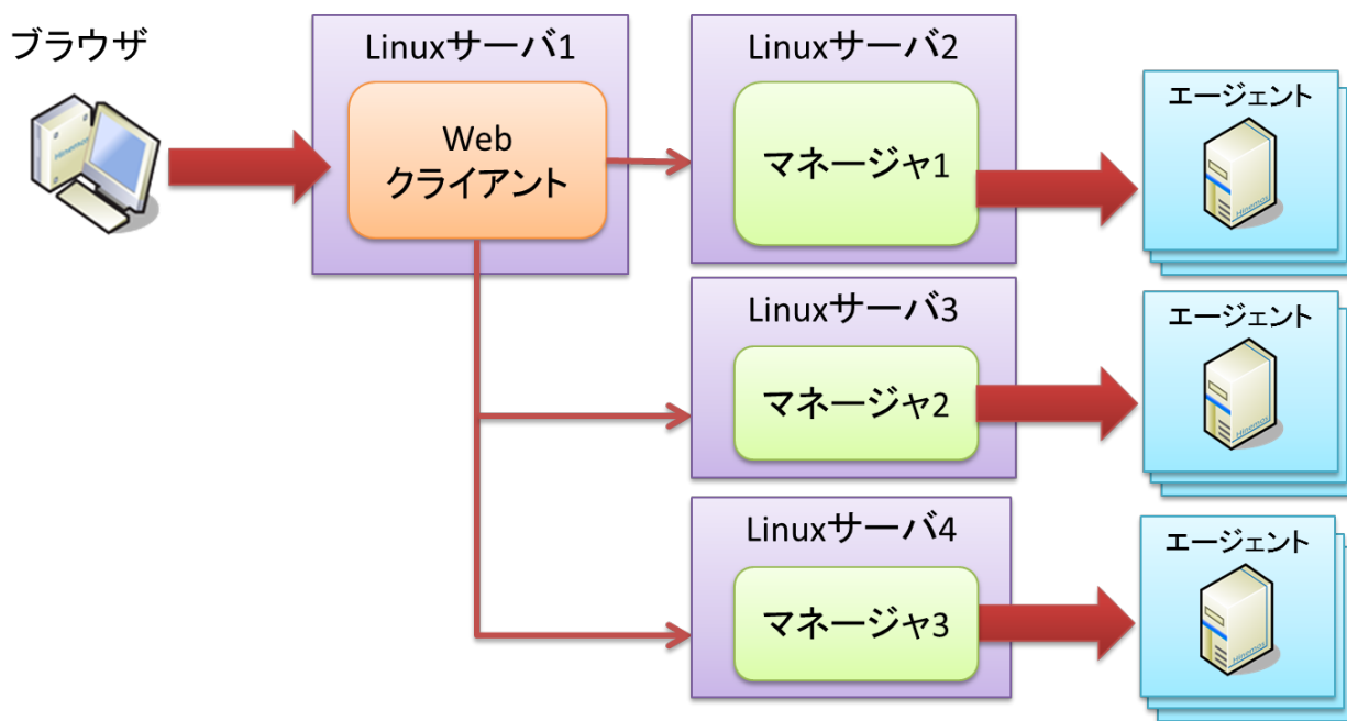
図 8-4 全体構成（Webクライアント）マルチマネージャ接続時 ※Webクライアントとマネージャが別居
