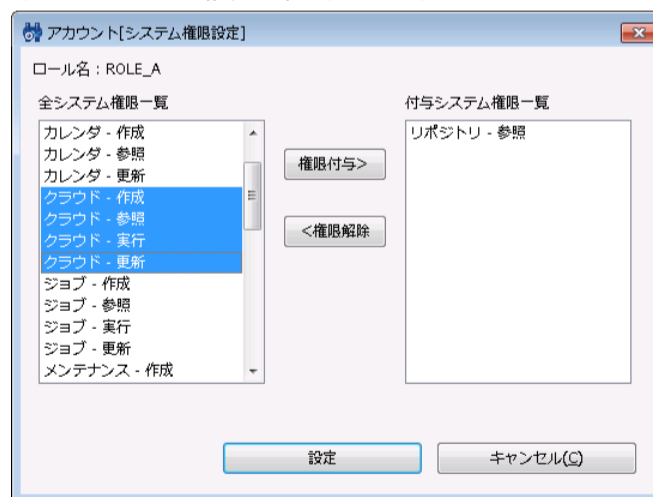
図4-1, アカウント[システム権限設定]ダイアログ(ロール作成時のデフォルト設定)
